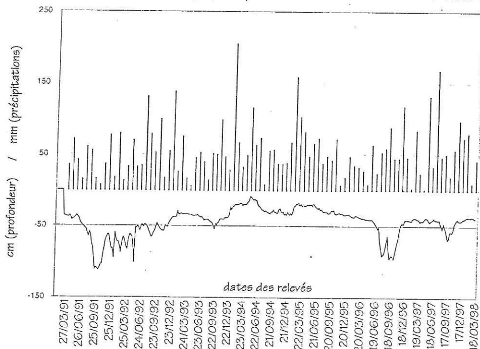
Exemple de représentation graphique d'un suivi piézométrique et pluviométrique Marais de la Souche (02) - d'après les données du Centre de Recherche de Cessières
