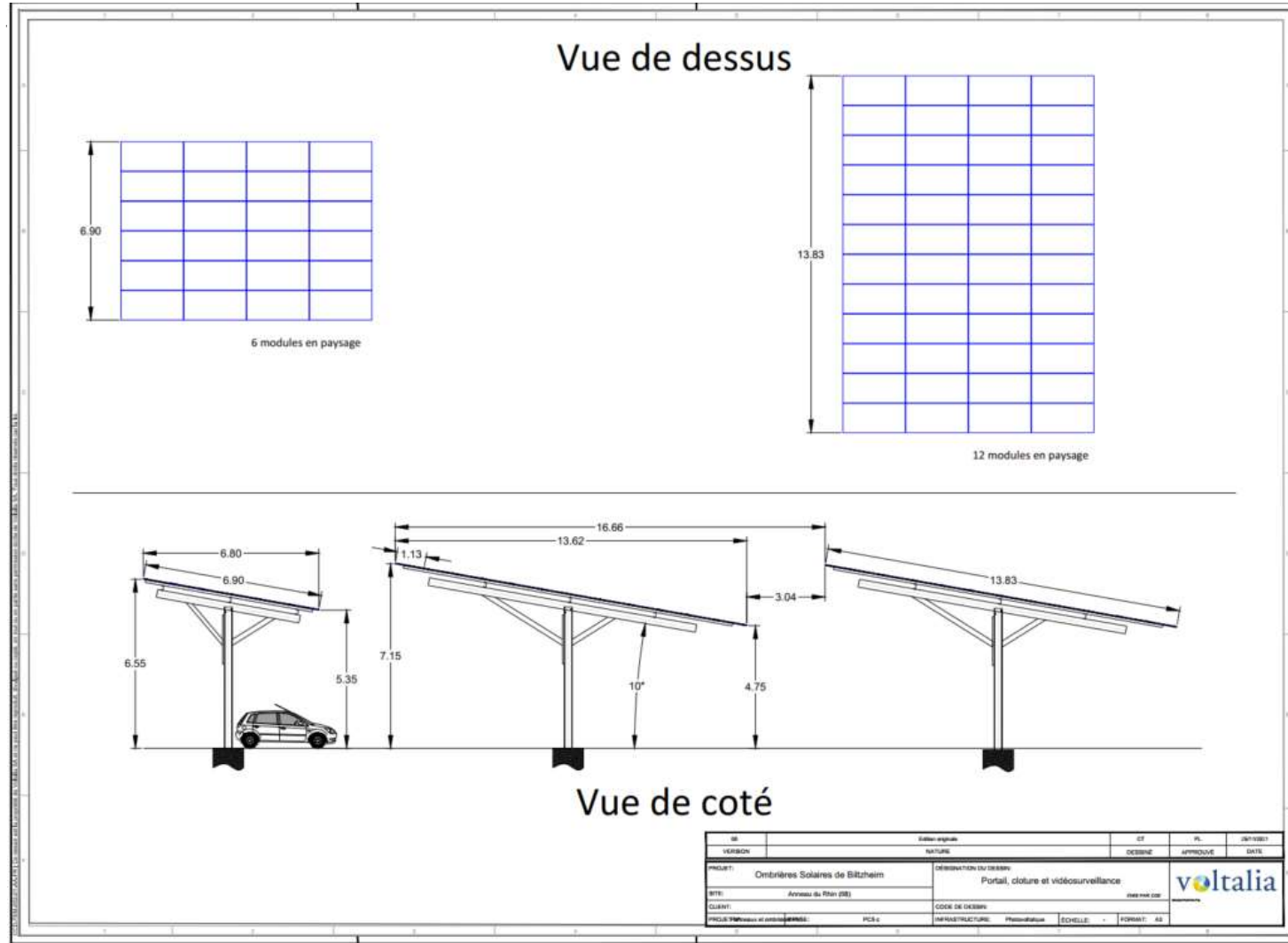
Plan de coupe d'une ombrière
