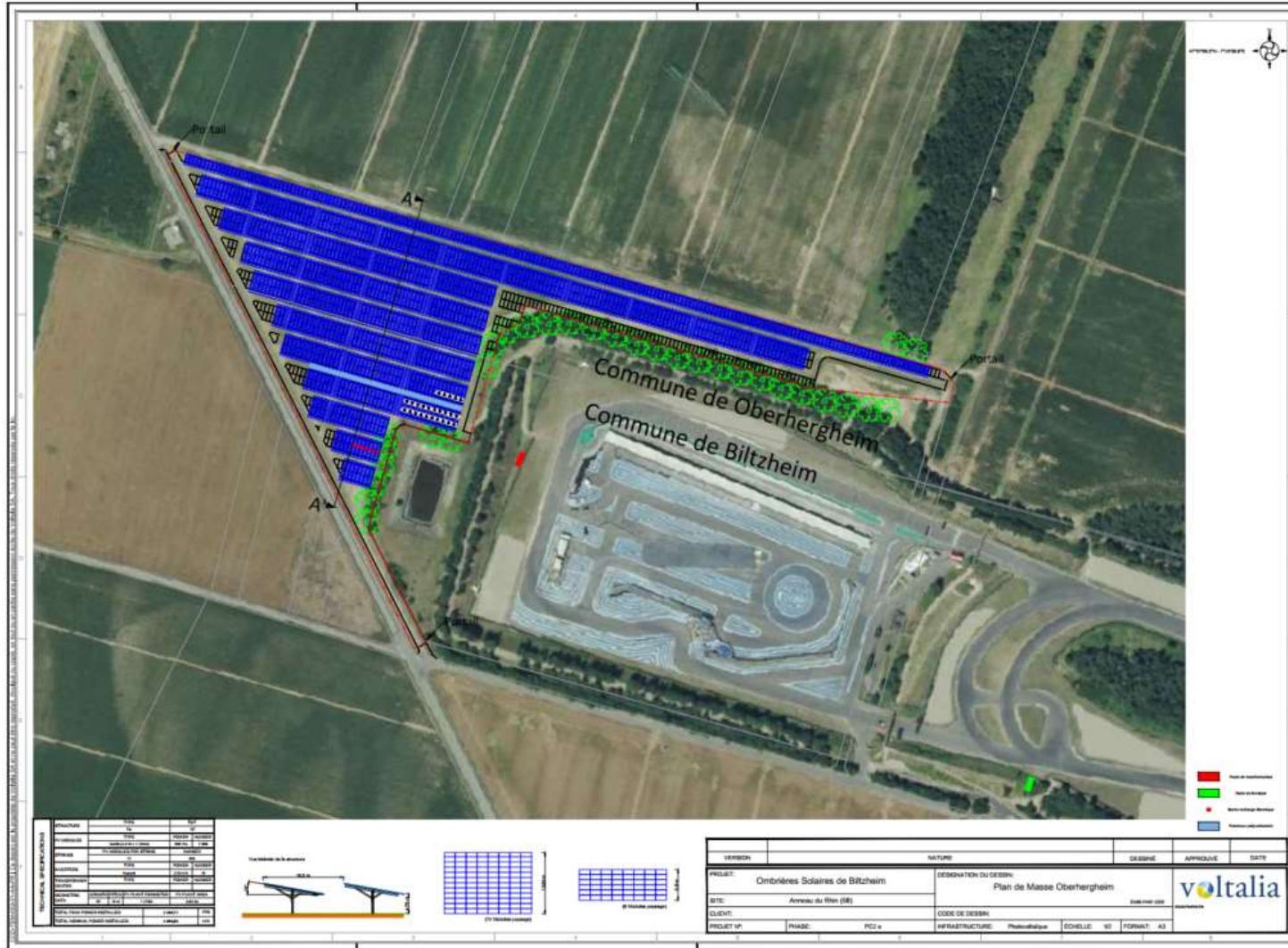
Plan de masse de l'opération
