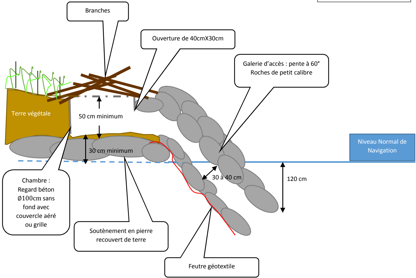
COUPE : vue de profil
