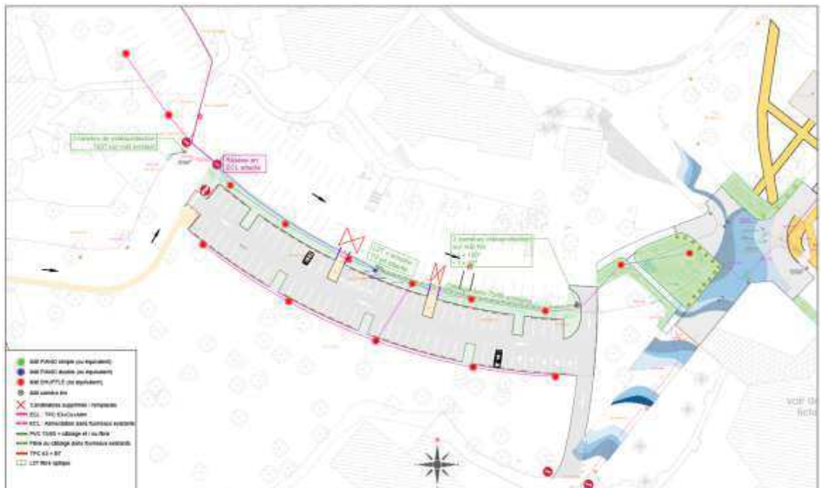
Fig. 4. Plan des réseaux secs - Parking centre 3
