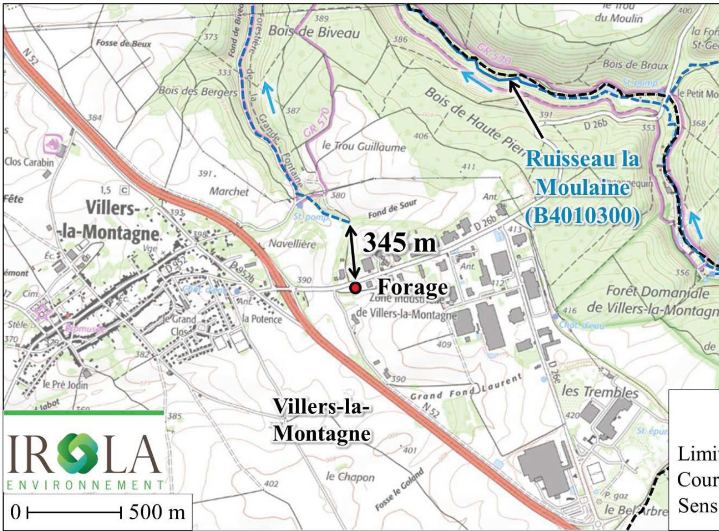
Annexe 8.1.2 : Plan de situation du forage de la commune de Villers-la-Montagne (Fond de carte topographique – Géoportail – Mai 2022)
