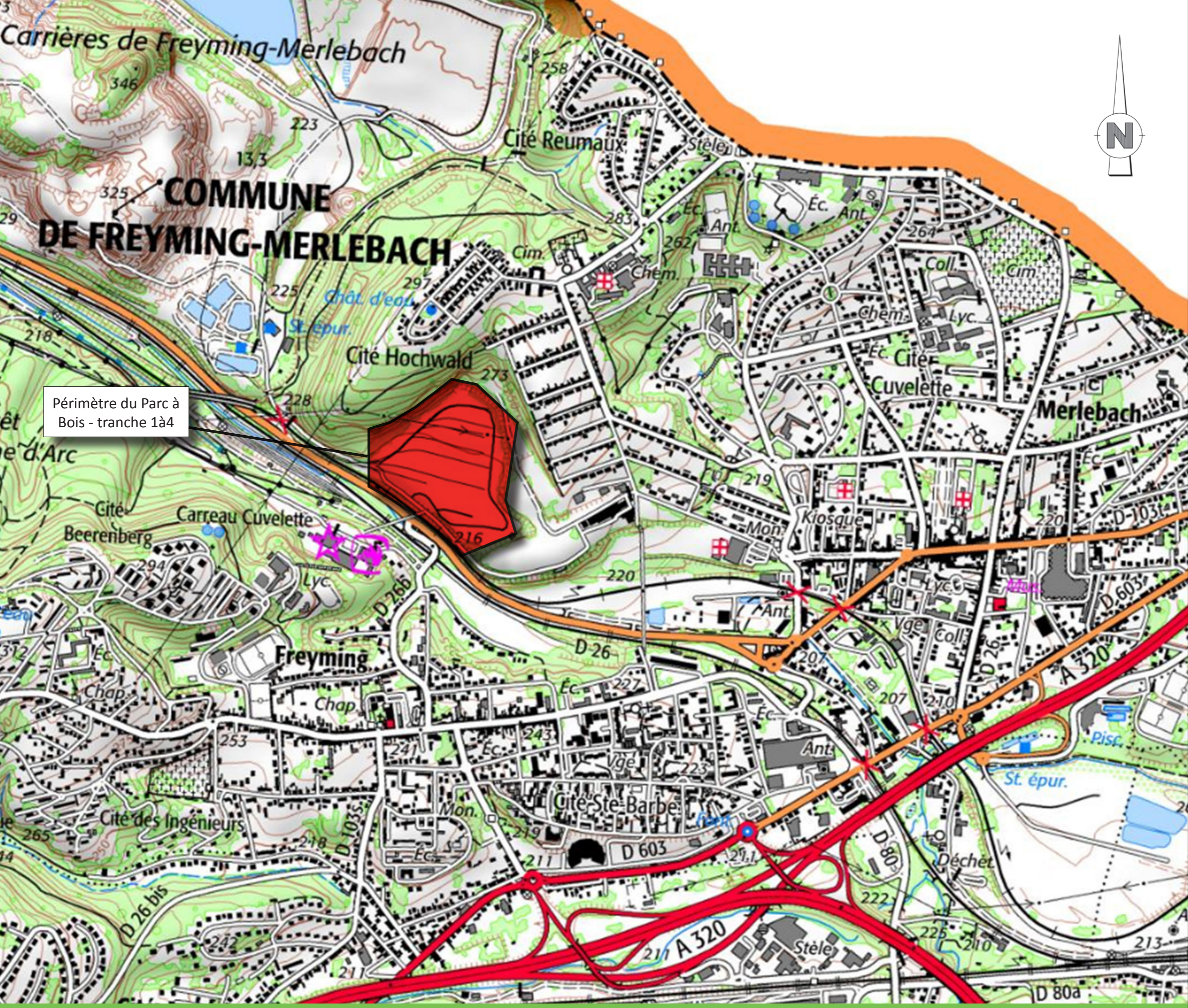
PA1. - PLAN DE SITUATION 1 : 20 000 e
