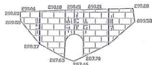
COUPE A Echelle 1/100
