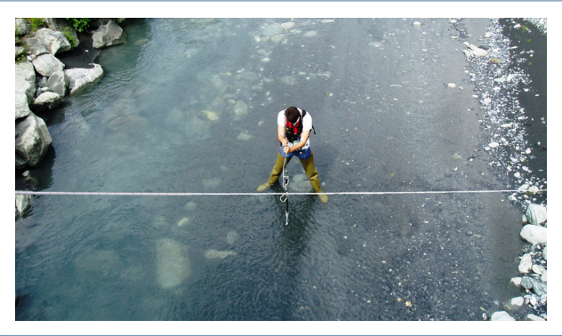
Jaugeage point par point à la perche (moulinet, courantomètre acoustique ou électromagnétique)
