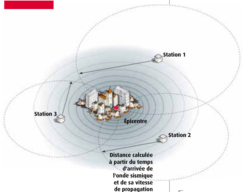
↖ Ci-contre , localisation de l'épicentre en fonction du temps d'arrivée des ondes sismiques
