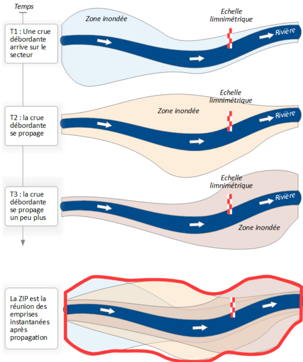
Figure 2: La ZIP est la représentation de l'enveloppe maximale de l'inondation durant sa propagation
