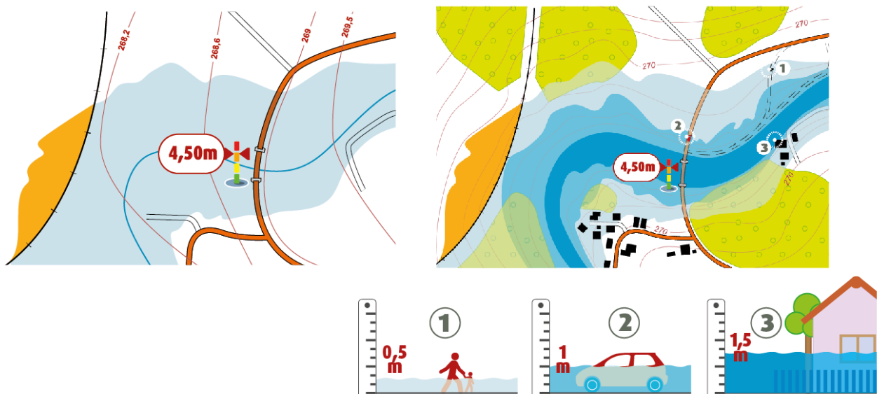
Figure 1: Schéma de principe des Zones d'Inondation Potentielle (ZIP), à gauche, et des Zones Inondées par Classes de Hauteurs d'eau (ZICH), à droite.
